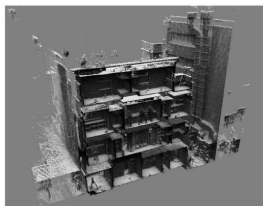
SLAM 技術を用いた構造物の三次元モデル
